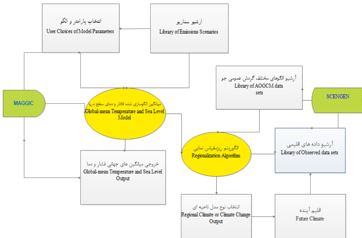
شکل ۱. الگوی MAGICC-SCENGEN در دو بخش Fig. 1. MAGICC-SCENGEN pattern in two sections
