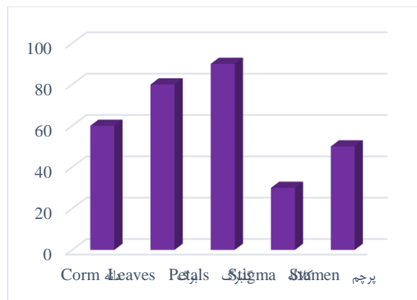
شکل ۳. بیان ژن DREB
