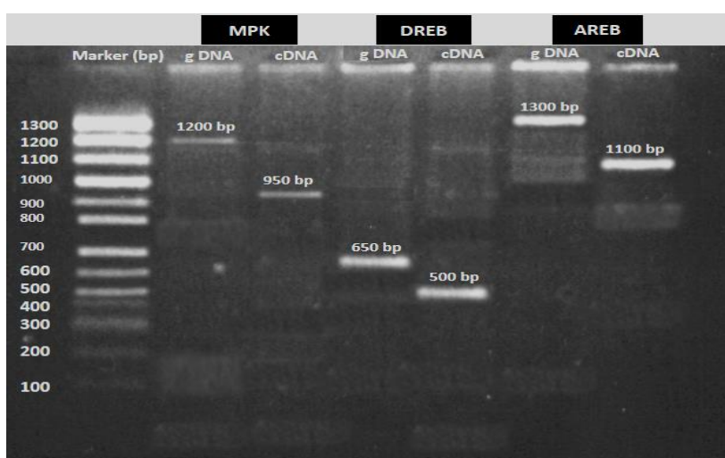
شکل ۱. ژل الکتروفورسز پس از PCR، قطعه ۱۳۰۰ و ۱۱۰۰، برای ژن AREB، قطعه ۶۵۰ و ۵۰۰، برای ژن DREB و قطعه ۱۲۰۰ و ۹۵۰، برای ژن MPK جفت بازی تکثیر شده به ترتیب از DNA ژنومی و cDNA
