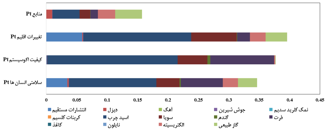
شکل ۶- سهم هریک از نهاده‌های ورودی در تولید مرغ گوشتی به روش صنعتی بر شاخص‌های نهایی وزن‌دهی شده زیست‌محیطی Figure 6. Contribution of inputs to broiler chicken production on weighted environmental indicators of the industrial method
