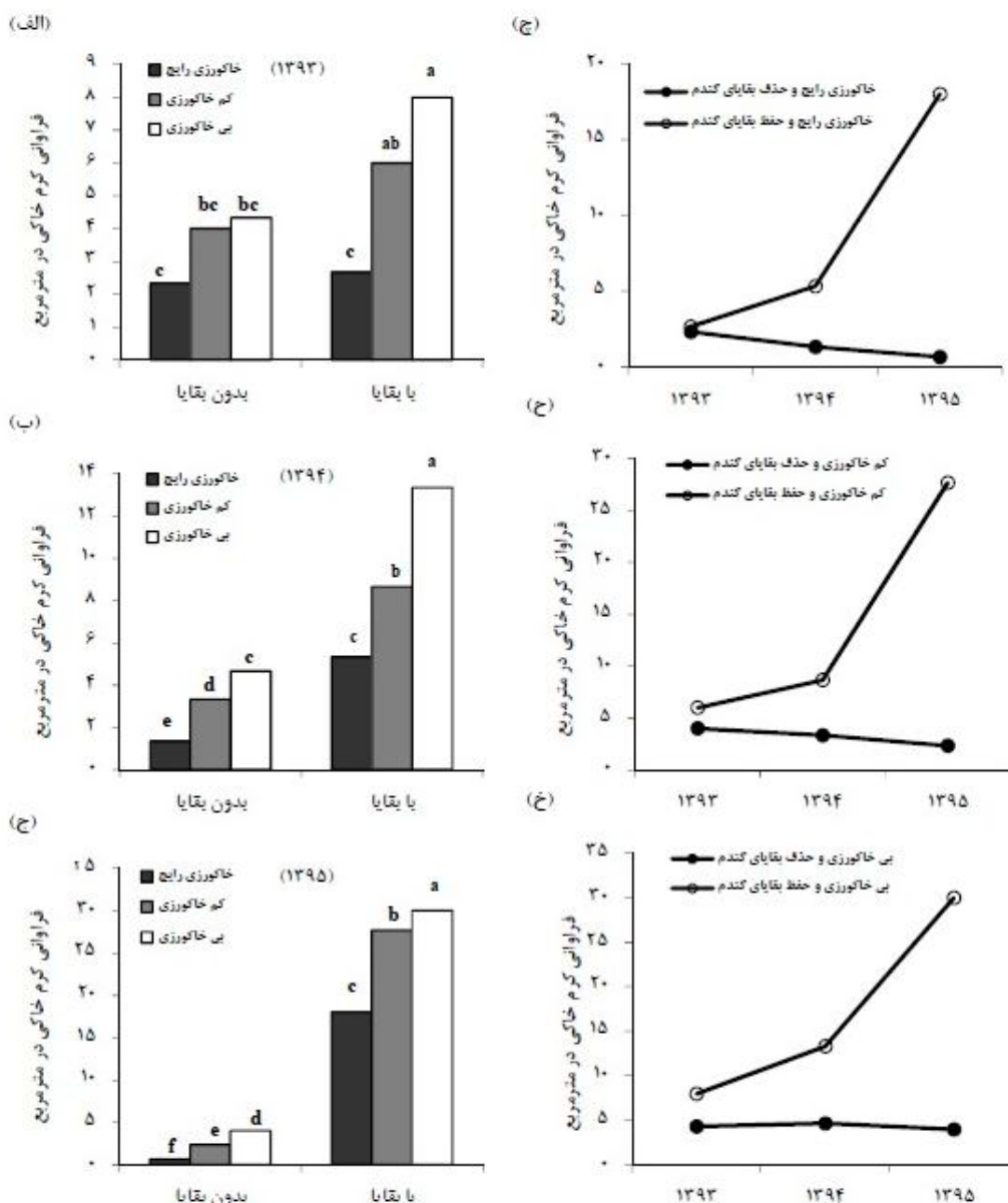
شکل 3- روند تغییرات کرم خاکی تحت تأثیر سامانه‌های خاک‌ورزی و مدیریت بقایای گندم در زمان پژوهش (ستون‌های با حروف مشابه بر اساس آزمون چند دامنه‌ای دانکن در سطح 5 درصد تفاوت معنی‌داری ندارند)
