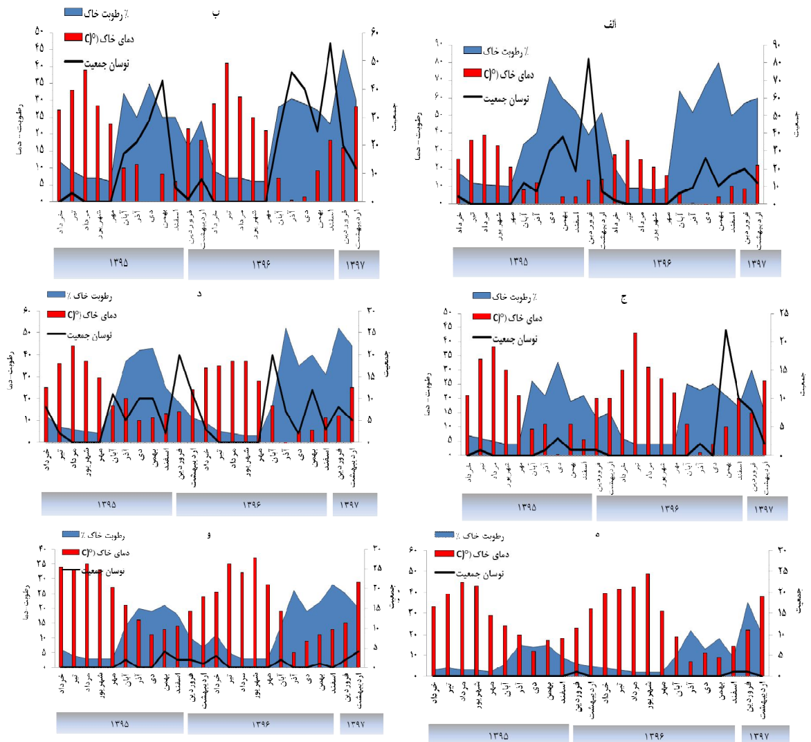
شکل 2- مقایسه فراوانی و نوسان جمعیت (از سطح 100 سانتی‌متر مربع و عمق 13 سانتی‌متر) گونه Folsomides marchicus در زیستگاه‌های مختلف شهرستان اسلام‌آباد غرب (الف، جنگل، ب) مرتع و (ج) مزرعه و گونه Pseudosinella octopunctata در زیستگاه‌های مختلف شهرستان سرپل‌دهاب (د، جنگل، ه) مرتع و (و) مزرعه
