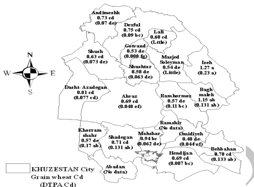
شکل ۳- مقادیر کادمیم بذر و قابل جذب (میلی گرم در کیلوگرم) در مناطق مورد مطالعه. Figure 3. Post map of total and DTPA-extractable Cd concentrations ( \text{mg.kg}^{-1} ) at different regions of the province.
