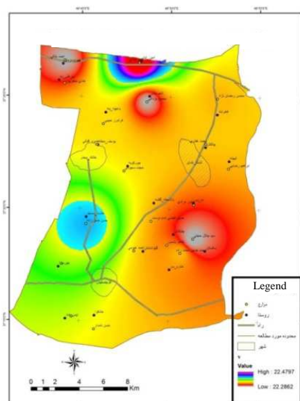
شکل ۴- میانگین تشعشع ورودی روزانه از کاشت تا گلدهی Figure 4. Mean daily shortwave radiation from planting to flowering
