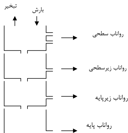
شکل ۲ دیاگرام مدل تانک ارائه شده توسط سوگوارا
