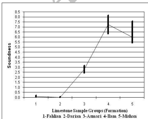
شکل (۷ و ۸) نمودار دامنه تغییرات مقاومت فشارشی تک محوری (خشک) و سلامت سنگ، سنگ‌های آهکی سازندهای مختلف منطقه
