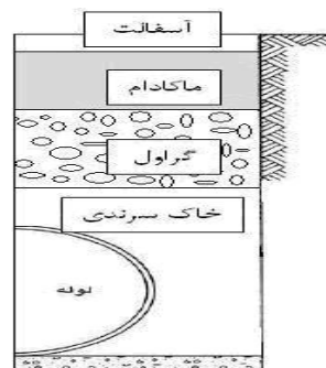
شکل(3): نیمه متقارن مقطع ترانشه و لوله مستقر در آن
