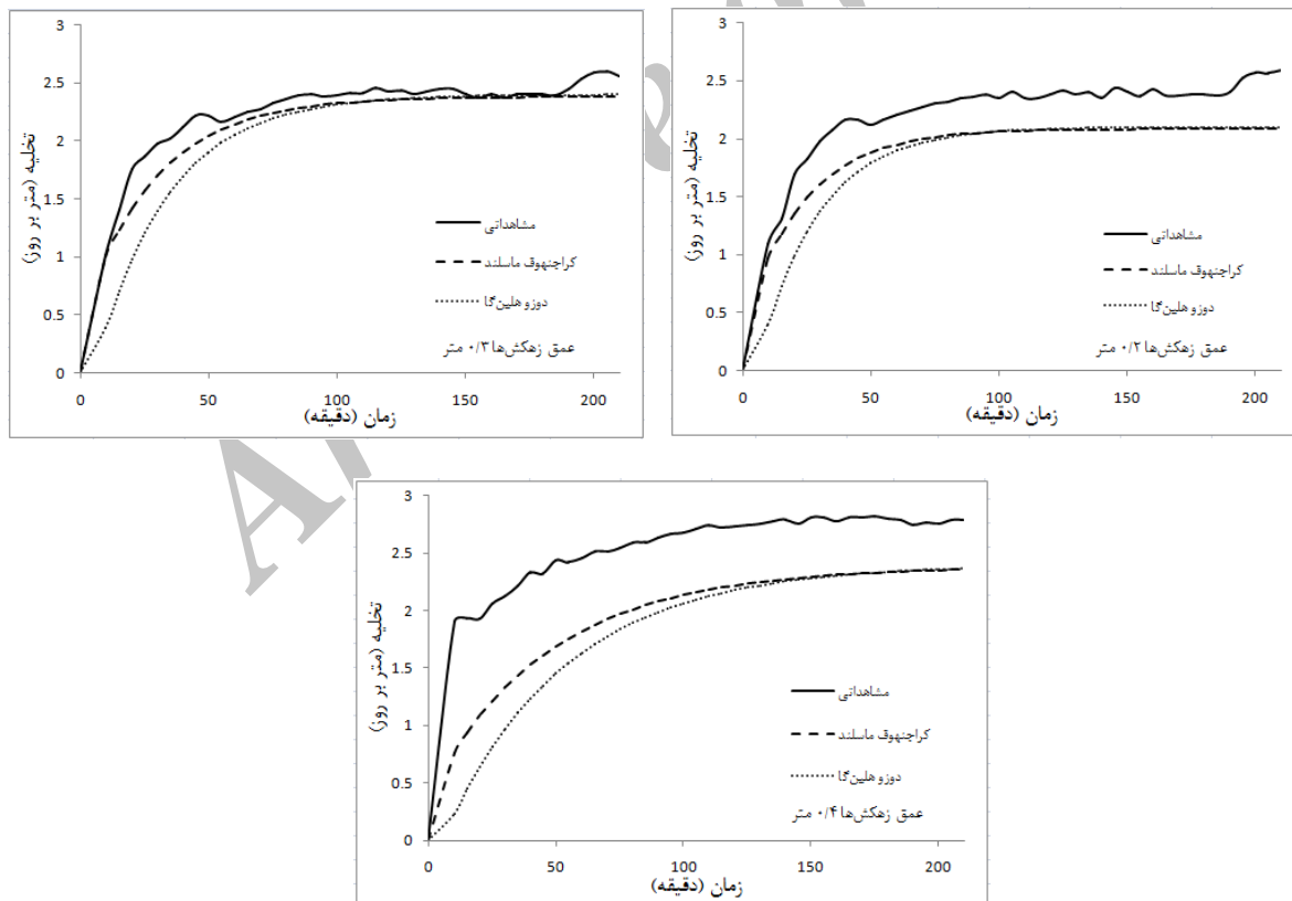
شکل (۳): تخلیه مشاهداتی و پیش‌بینی شده مدل‌های دوزو - هلین‌گا و کراجنهوف وان دلور - ماسلند در سطح ایستابی خیزان
