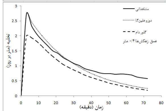
شکل (۵): مقادیر تخلیه مشاهداتی و پیش‌بینی شده توسط مدل‌های دوزو - هلین‌گا و گلور - دام در سطح ایستابی افتان
