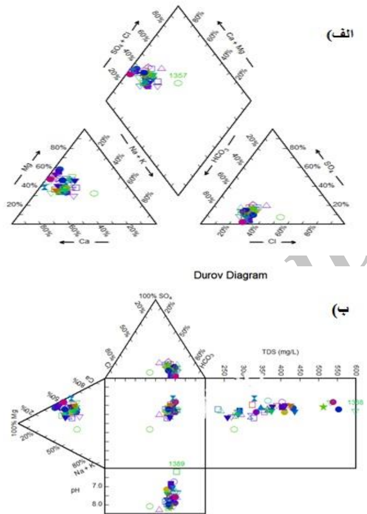
شکل (۳): نمودار پایپر (الف) و نمودار دروو (ب) مربوط به پارمترهای کیفیت آب رودخانه چم انجیر خرم آباد
