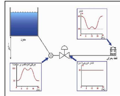
شکل (۳): مدیریت فشار با فشارشکن خروجی ثابت (وزارت نیرو ۱۳۸۶)
