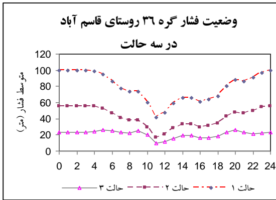
شکل (۱۲): نمودار فشار در گرہ ۳۶ روستای قاسم آباد در سه حالت
