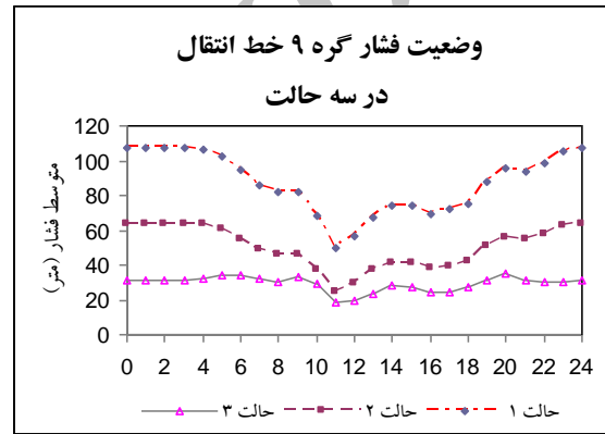
شکل (۱۱): نمودار فشار در گرہ ۹ از خط انتقال در سه حالت
