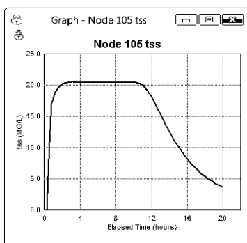
شکل (۴): کاهش غلظت جامدات معلق در سناریو ۴
