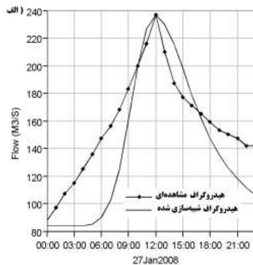
شکل (۴): مقایسه هیدروگراف مشاهده‌ای و شبیه سازی الف) در مرحله واسنجی حوضه قرنقو در تاریخ ۸۴/۱/۲۷ و ب) در مرحله صحت‌سنجی حوضه قرنقو در تاریخ‌های ۸۴/۲/۲۵ و ۸۴/۲/۲۶
