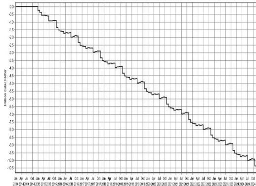
شکل (۸): نسبت تغییرات حجم مخزن آب زیرزمینی در سناریوی خشک‌سالی در مقایسه با سناریوی مرجع
