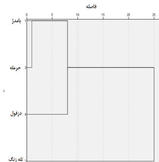
شکل (۳): نمودار دندوگرام حاصل از تحلیل خوشه‌ای
