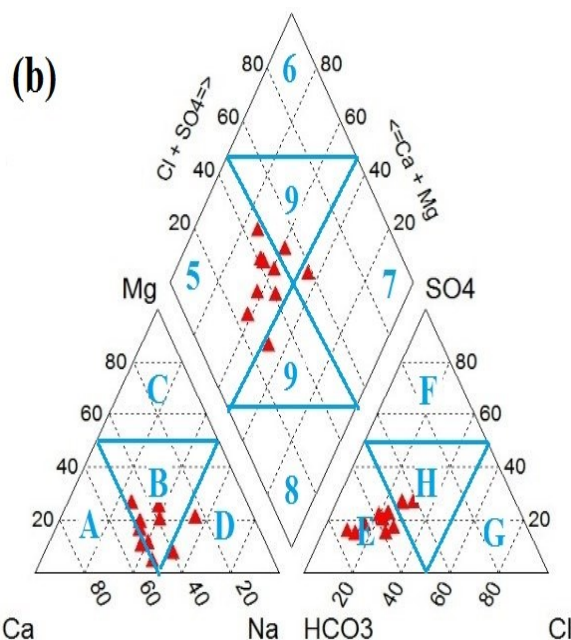
شکل (۵): نمودار پایپر برای تعیین تیپ بندی آب در منطقه (a) نمودار پایپر برای تیپبندی چاه‌های ۱ تا ۳ و شکل (b) نمودار پایپر برای تیپبندی آب رودخانه آبدانان در منطقه مورد مطالعه
