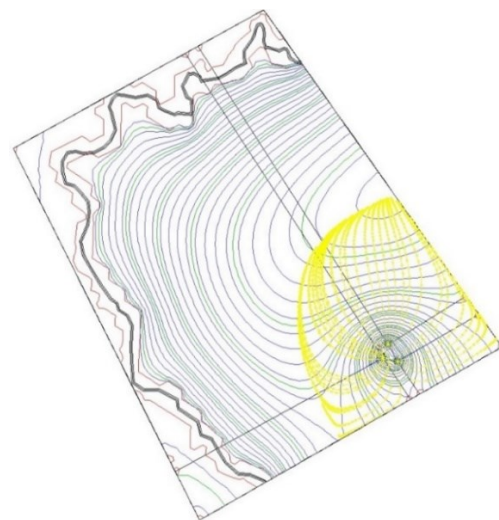
شکل (۷) : نحوه جریانات هیدرولیکی در آبخوان جریانات ناشی از رودخانه در آبخوان قبل از برداشت آب از چاهها
