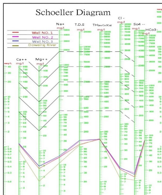
شکل (۴): نمودار شولر برای چاه‌های مورد منطقه
