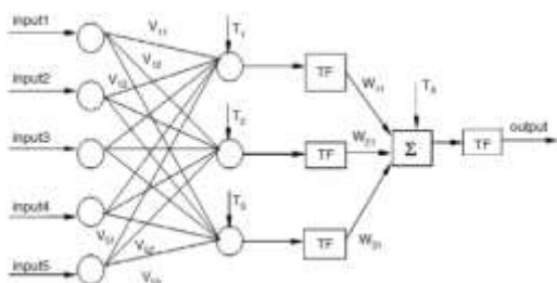
شکل ۶ ساختار شبکه عصبی مصنوعی چند لایه برای پیش بینی دبی کانال مرکب (Sahu et al., 2011)
