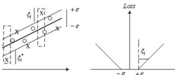
شکل ۴ تنظیمات کمترین حاشیه نرم برای SVM خطی و تابع کاهش شدت اِپسِیلین (Wang et al., 2009).
