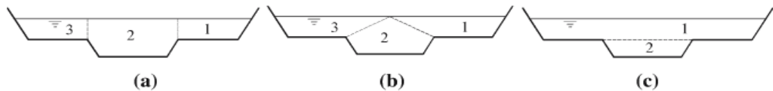
شکل ۲: انواع تقسیم‌بندی کانال مرکب. (a) تقسیم‌بندی بروش عمودی (Vertical)، (b) تقسیم‌بندی بروش قطری (Diagonal)، (c) تقسیم‌بندی بروش افقی (Horizontal) (Sahu et al., 2011).
