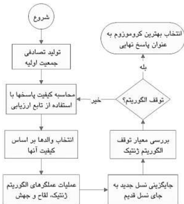
شکل (۱): چارت الگوریتم ژنتیک در پژوهش حاضر
