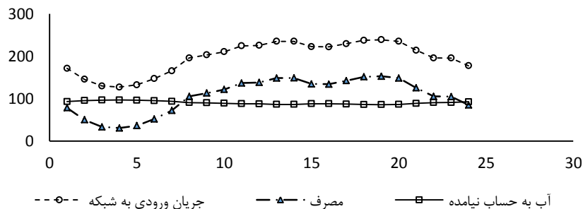
شکل ۶: تغییرات مصرف، نشت و آب به حساب نیامده مشترکین در شبکه
