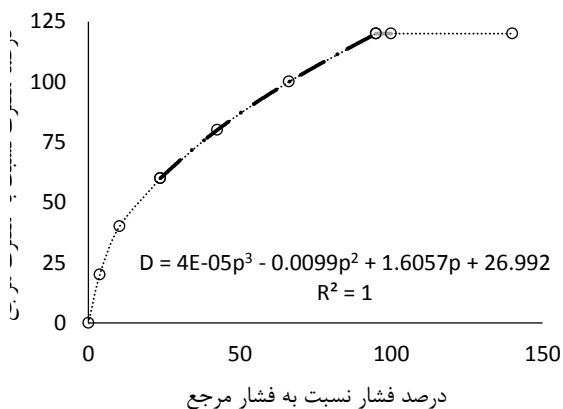
شکل ۱: رابطه مصرف با فشار
