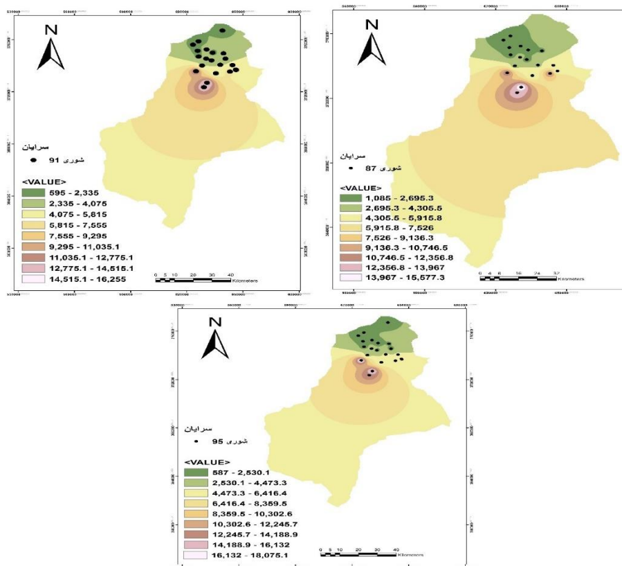
شکل (۷): تغییرات مکانی شوری (میکروموس بر سانتیمتر)
