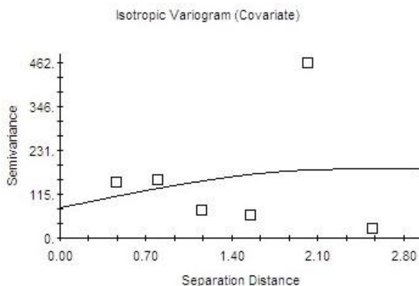
شکل ۳- واریوگرام متغیر کمکی (رطوبت مطلق حداکثر) با مدل کروی
