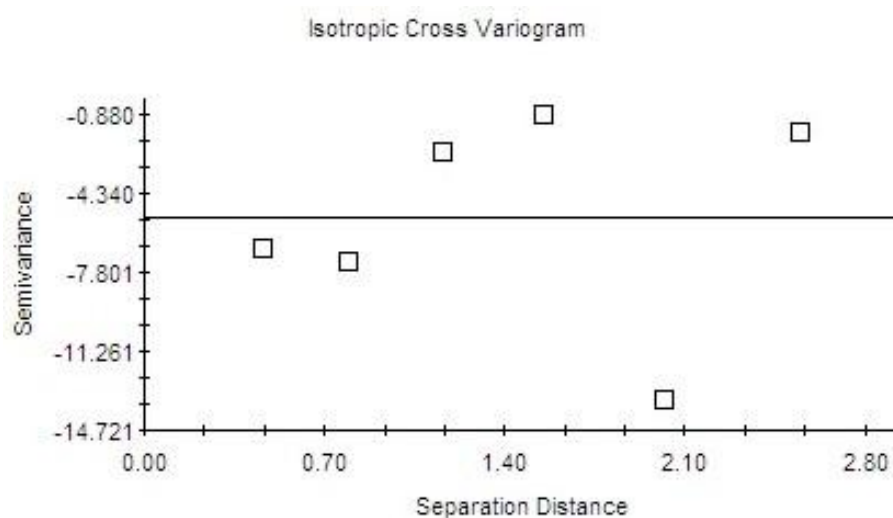
شکل ۴- واریوگرام متقاطع متغیرهای اصلی و کمکی با مدل خطی
