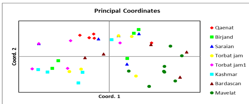
شکل ۲- نمودار دو بعدی تجزیه به مختصات اصلی ارتباط ژنتیکی جمعیت‌های A. alternata
