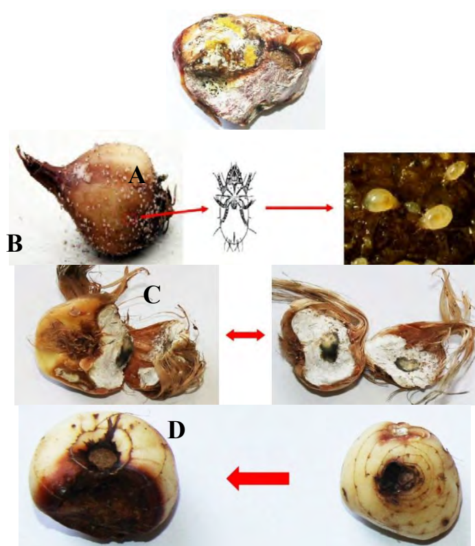
شکل ۲- نمونه‌هایی از علائم شایع ناشی از آسیب‌های فیزیکی، فعالیت آفات و عوامل بیماری‌زا در بنه‌های زعفران A: بیماری سفیدک سطحی که ممکن است در اثر بروز صدمات فیزیکی به بنه‌ها در زمان برداشت شدیداً گسترش یابد؛ B: کنه بنه زعفران ( Rhizoglyphus robini )؛ C: پوسیدگی بنه زعفران ( Penicillium digitatum )؛ D: پوسیدگی نکرزه بنه ( Rhizoctonia crocorum )
