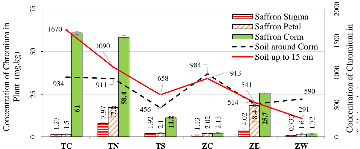
شکل ۶- غلظت کروم در گیاه زعفران و خاک مزارع زعفران (غرب زاوه: ZW، شرق زاوه: ZE، مرکز زاوه: ZC، جنوب تربت حیدریه: TS، شمال تربت حیدریه: TN، مرکز تربت حیدریه: TC)
