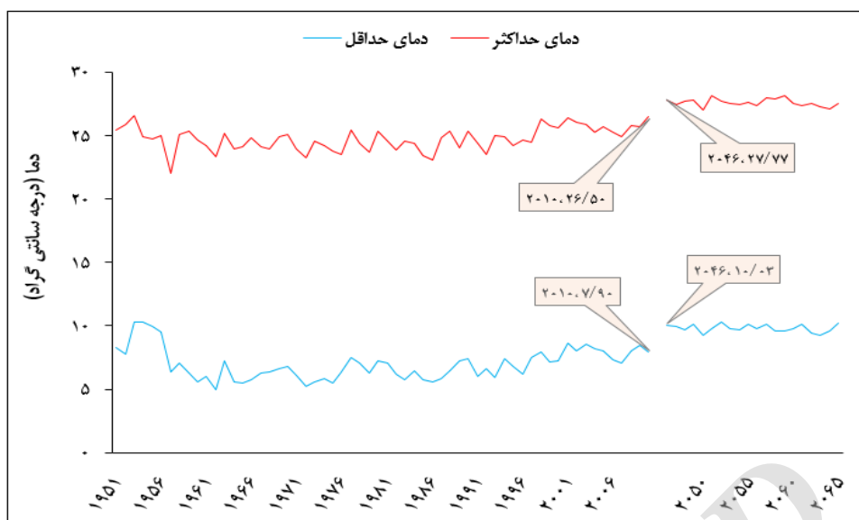
شکل ۷- تغییرات دمای کمینه و بیشینه سالانه دوره آینده (۲۰۴۶-۲۰۶۵) نسبت به دوره پایه (۲۰۱۰-۱۹۵۱)
