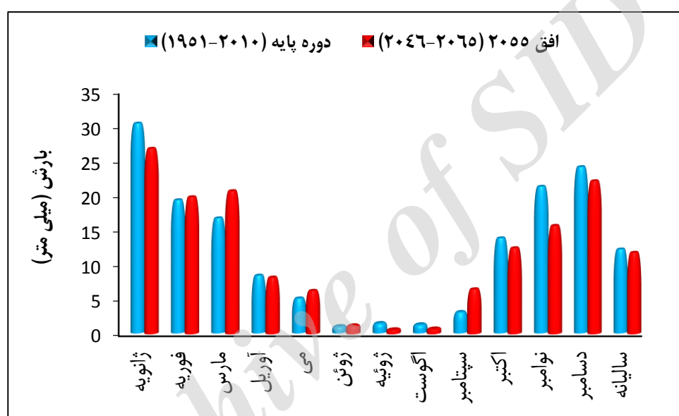
شکل ۲- مقایسه بارش ماهانه و سالانه برای دوره پایه (۲۰۱۰-۱۹۵۱) و افق (۲۰۴۶-۲۰۶۵)
