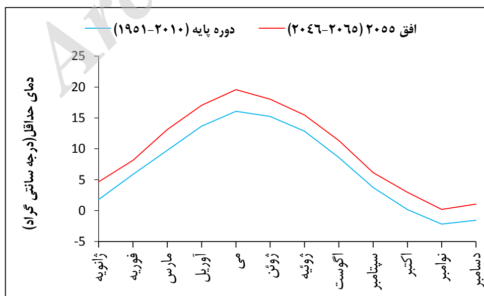
شکل ۳- مقایسه دمای کمینه ماهانه برای دوره پایه (۲۰۱۰-۱۹۵۱) و افق (۲۰۴۶-۲۰۶۵)
