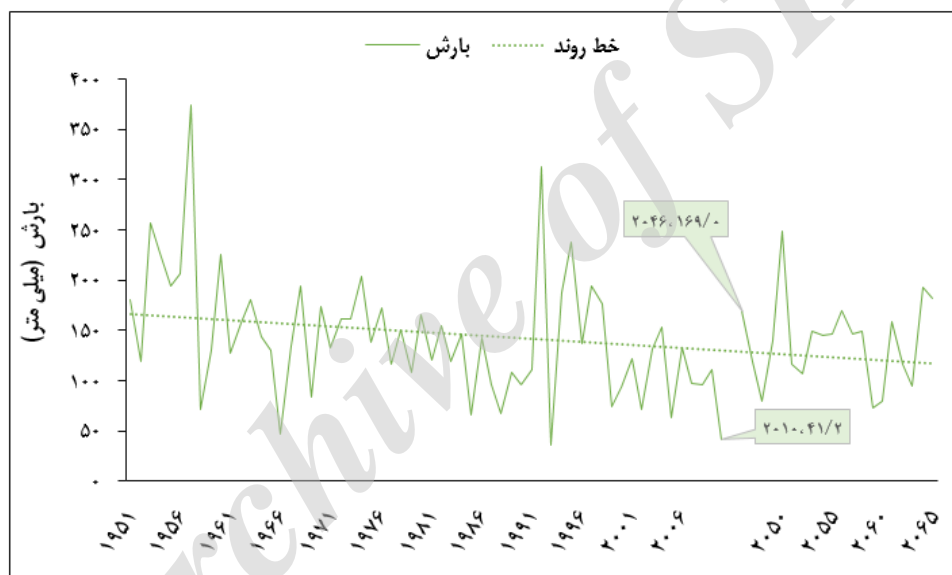
شکل ۸- تغییرات بارش سالیانه دوره آتی (۲۰۴۶-۲۰۶۵) دشت کرمان-باغین نسبت به دوره پایه (۲۰۱۰-۱۹۵۱)
