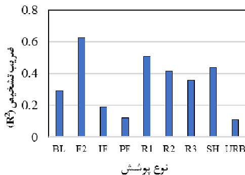
شکل 11- میانگین مقدار همبستگی شاخص خشکسالی SPI 12 ماهه و شاخص NDVI فصل بهار (چپ) و فصل تابستان (راست) در پوشش‌های مختلف
