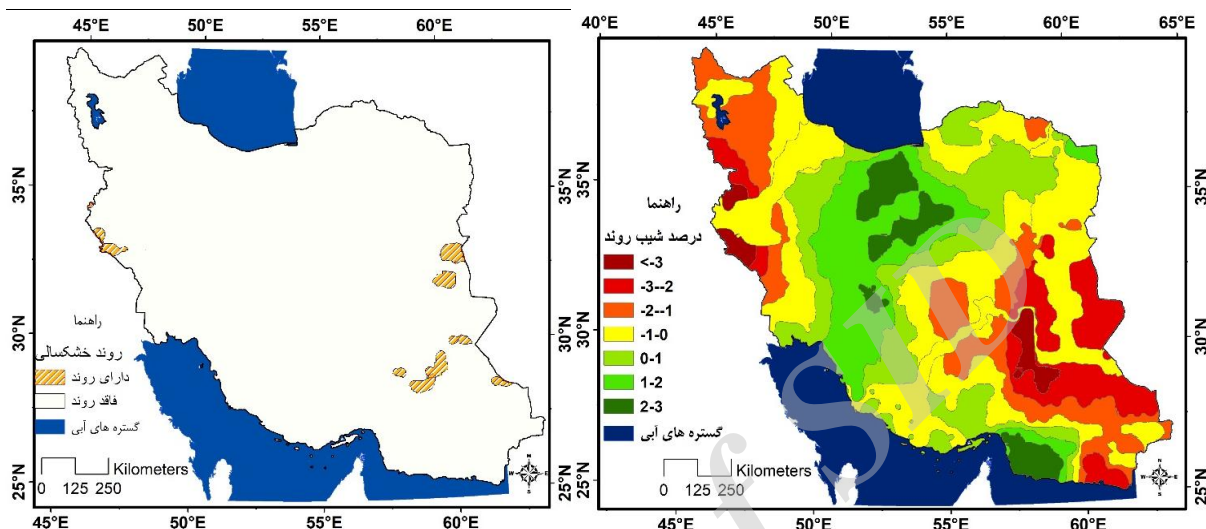
شکل 4. وضعیت روند (شکل سمت چپ) و شیب خط روند (شکل سمت راست) خشکسالی در فصل پاییز
