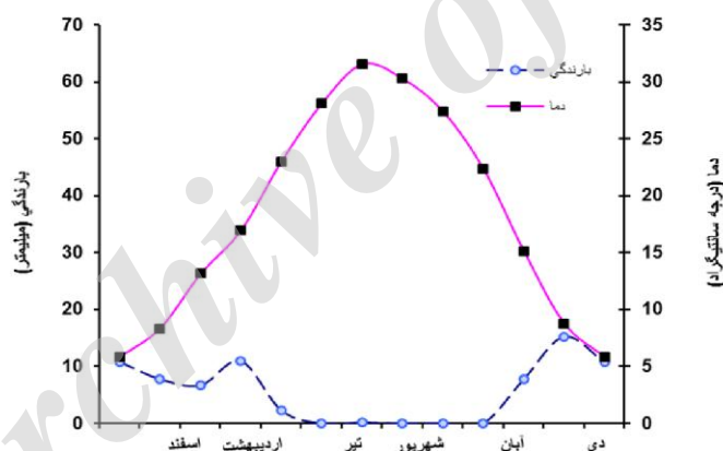
شکل 2. منحنی آمبروترمیک ایستگاه هواشناسی مهریز طی سال‌های 1380-1395
