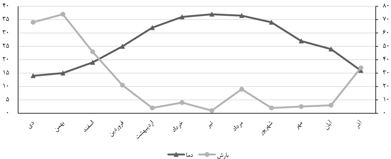
شکل ۳. منحنی آمبروترمیک ایستگاه هم‌دیدگی کهنوج
