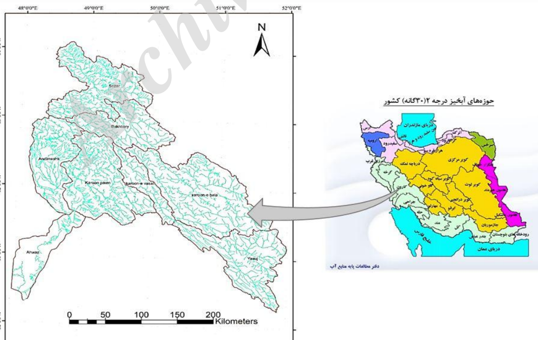
شکل ۱. موقعیت حوضه آبخیز کارون
