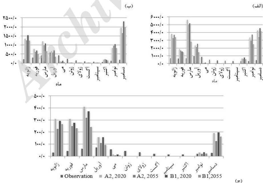
شکل ۵. متوسط درازمدت دبی ماهانه (مترمکعب بر ثانیه) در زیرحوضه الف) اهواز، ب) اندیمشک و ج) یاسوج برای دوره های آتی و پایه
