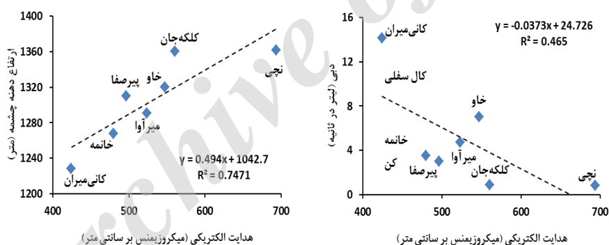
شکل ۲. ارتباط دبی و ارتفاع دهانه چشمه‌ها با میزان هدایت الکتریکی آنها در منطقه پژوهش‌شده
