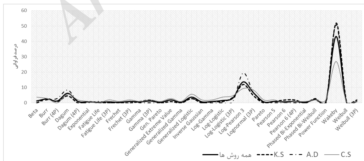
شکل 2. نمودار درصد فراوانی توزیع‌های منتخب در ایستگاه‌های بررسی شده با استفاده از آزمون‌های نکویی برازش
