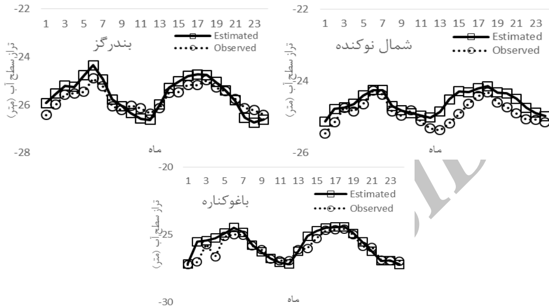
شکل ۳. نمودار سری زمانی تراز سطح آب زیرزمینی مشاهداتی و محاسباتی در نوار ساحلی آبخوان بندرگز
