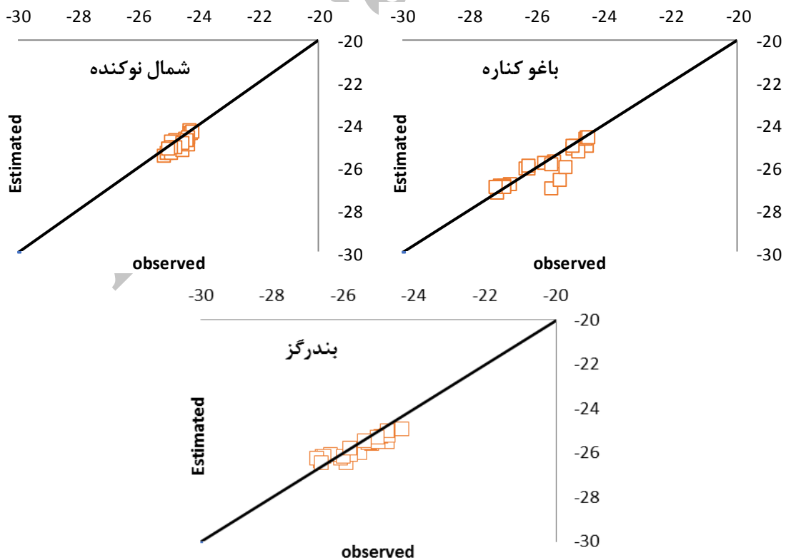
شکل ۴. نمودار خط ۴۵ درجه مقایسه تراز سطح آب زیرزمینی مشاهداتی و محاسباتی در نوار ساحلی آبخوان بندرگز
