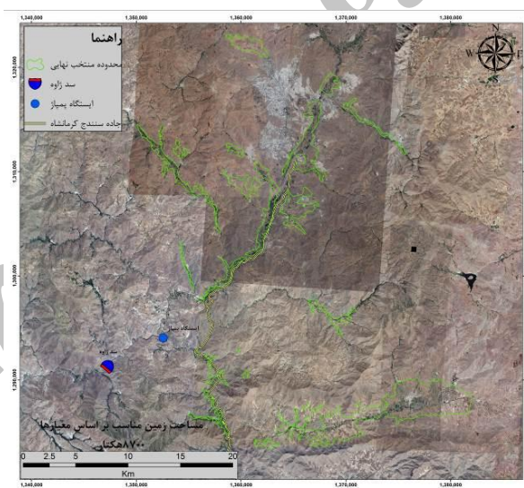
شکل ۱۶. نقشه محدوده منتخب نهایی - حالت سوم: ۴۰۰ متر پمپاژ
