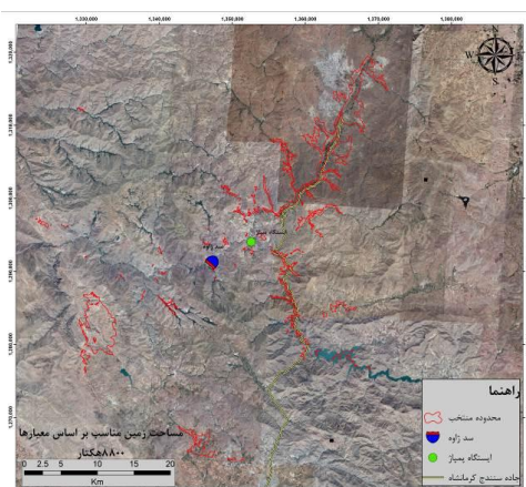
شکل ۱۴. محدوده منتخب - حالت دوم: ۲۰۰ متر پمپاژ
