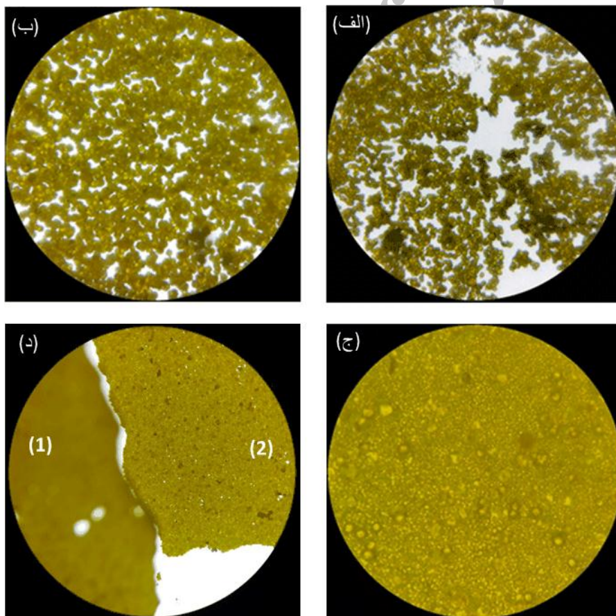
شکل ۵. تصاویر میکروسکوپ نوری برای لایه‌های \text{BiVO}_4 آماده‌شده در غلظت‌های مختلف پیش‌ماده الف) نمونه 9mM ب) نمونه 18mM، ج) نمونه 27mM و د) نمونه 36mM بخش جداشده از سطح FTO و ۲. بخش متصل به FTO
