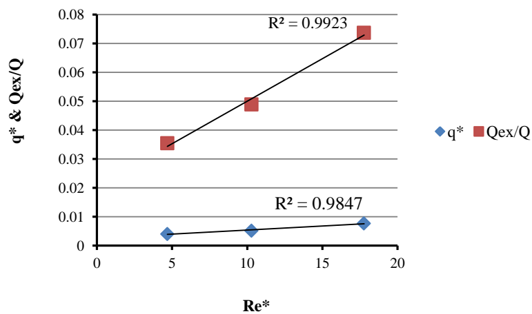
شکل ۱۰. مقادیر بی بعد دبی تبدالی و درصد دبی تبدالی در مقابل رینولدز جریان زیرسطحی
