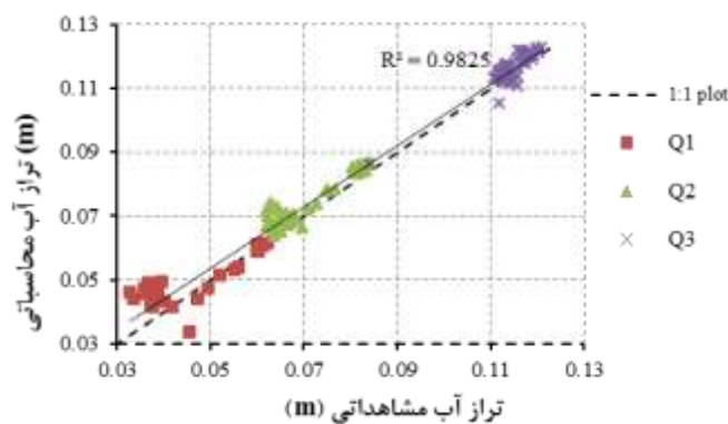
شکل ۴. نمودار مقادیر مشاهداتی و محاسباتی تراز آب برای کل داده‌ها
