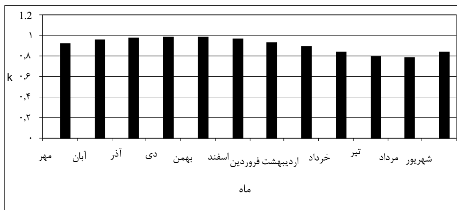
شکل ۲. وضعیت تغییرات ثابت کاهش رطوبت خاک در ماه‌های مختلف در حوضه کارده
