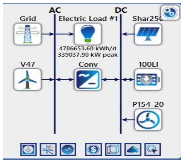
شکل ۷. پیکربندی سیستم هیبریدی تجدیدپذیر شبیه‌سازی‌شده توسط نرم‌افزار هومر
