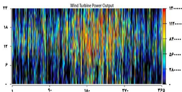
شکل ۹. میزان توان خروجی توسط توربین‌های بادی طی روز
