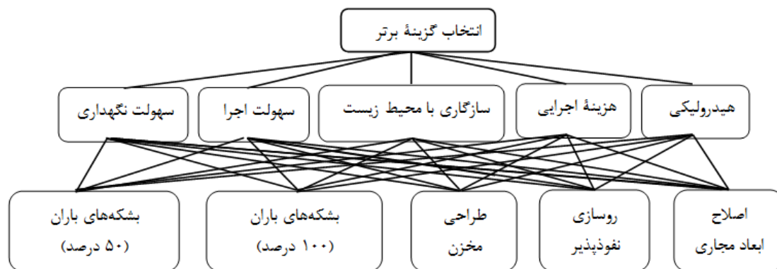
شکل ۸. ساختار سلسله‌مراتبی
