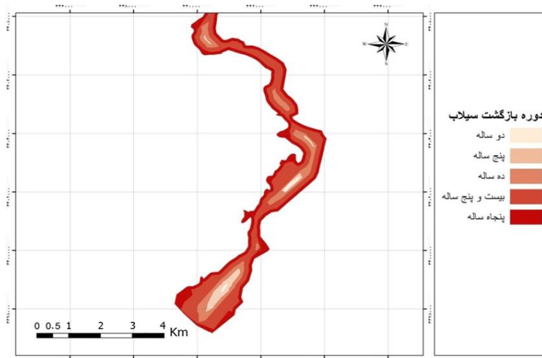
شکل ۱۱. نقشه پهنه‌بندی سیلاب با دوره بازگشت‌های مختلف در رودخانه مارون
