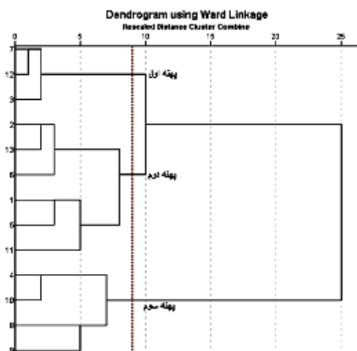
شکل (۱): نمودار درختی احتمال شرطی حالات بارش به شرط حالات دمایی در استان فارس
