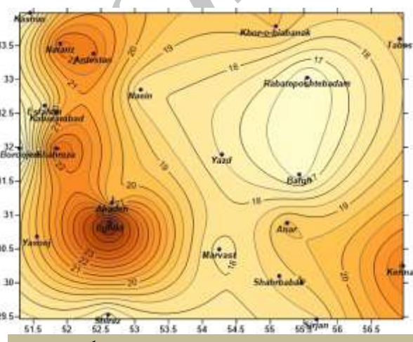
شکل (۳): بیشینه سرعت باد (متر بر ثانیه) در دوره بازگشت ۲ ساله
