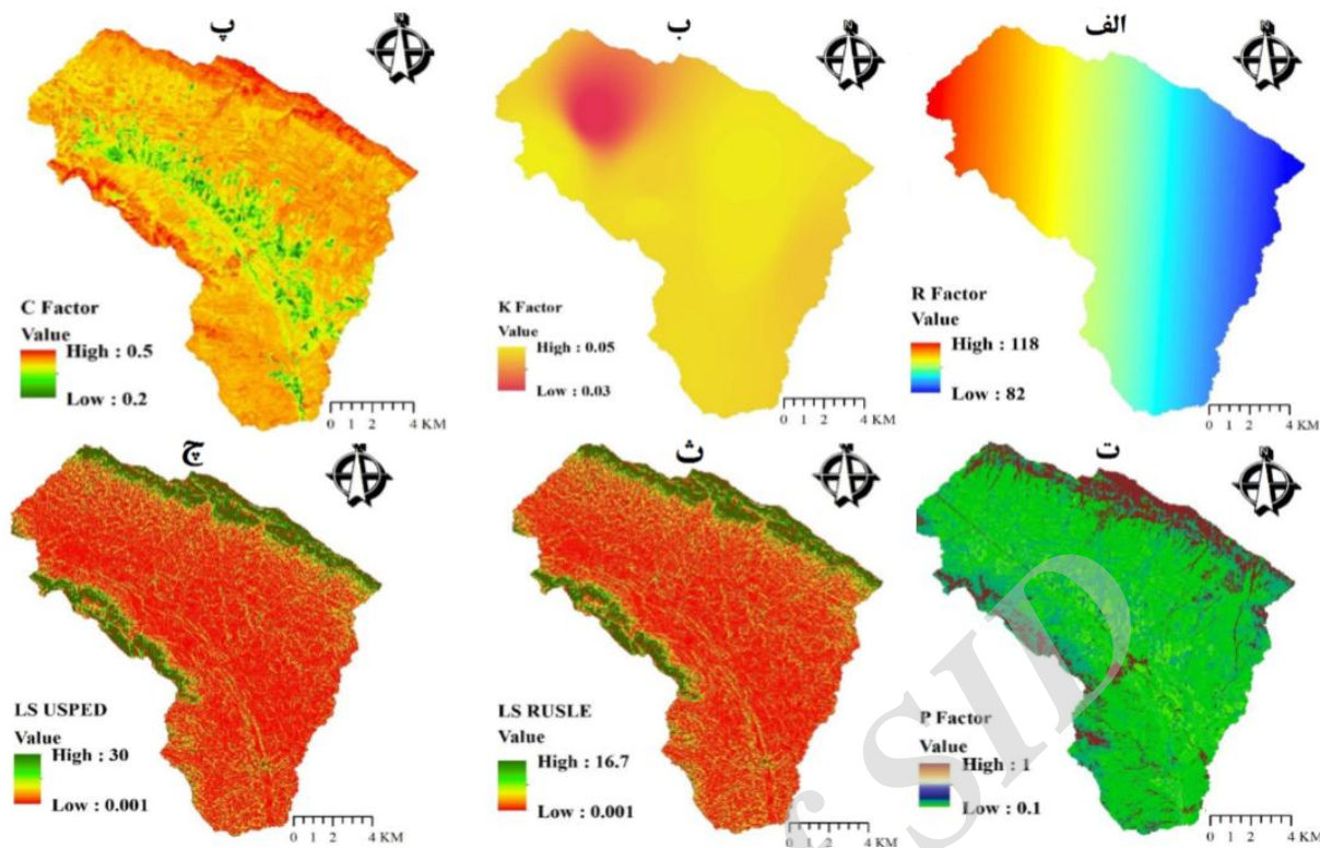
شکل (۲): الف. عامل فرسایش‌دگی ( \text{MJ mm ha}^{-1} \text{y}^{-1} \text{h}^{-1} )، ب. عامل فرسایش‌پذیری ( \text{t h MJ}^{-1} \text{mm}^{-1} )، پ. عامل مدیریت پوشش گیاهی،
