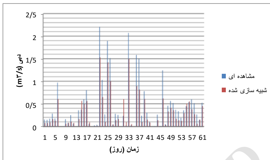
شکل (۶): مقادیر دبی مشاهده‌ای و شبیه‌سازی‌شده در زمان پوشش ابر کومولونیمبوس Figure (6): Observed and simulated discharges during cumulonimbus clouds
