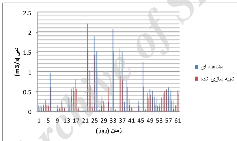
شکل (۷): مقادیر دبی مشاهده‌ای و شبیه‌سازی‌شده در زمان پوشش ابر استراتوکومولوس Figure (7): Observed and simulated discharges during stratocumulus clouds
