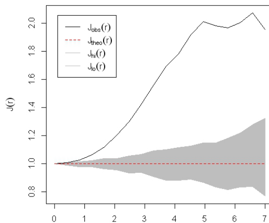
شکل ۵. شاخص J(r) درختان بلوط ایرانی در منطقه مورد مطالعه
