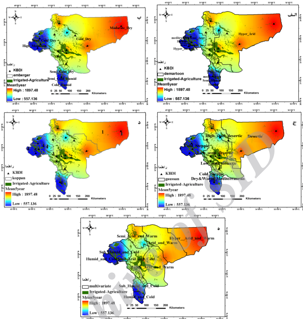
شکل ۲. نقشه پهنه‌بندی اقلیمی شاخص خشکی کچ-بایرام با دوره آماری ۵ ساله در استان آصفهان بوسیله طبقه‌بندی اقلیمی دومارتن (الف)، آمبرژه (ب)، گوسن (ج)، کوپن (د)، چند متغیره (ه)
