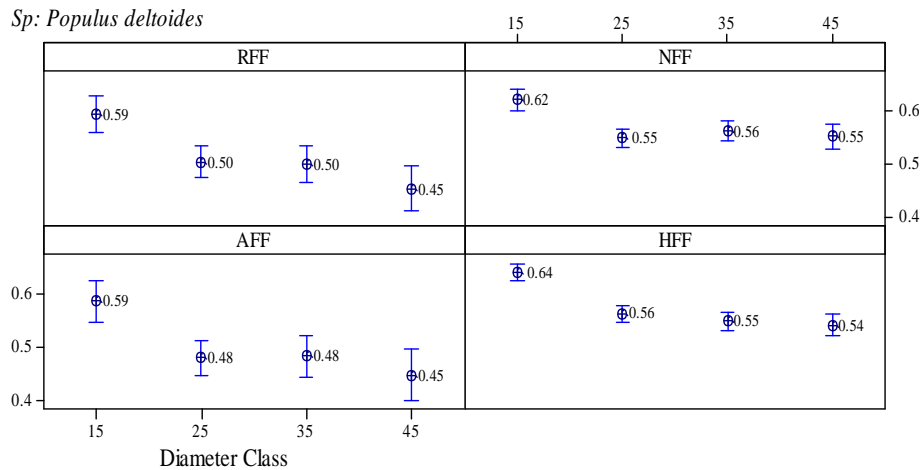
شکل ۴. تغییرات در طبقات قطری روش‌های واقعی (RFF)، طبیعی (NFF)، مصنوعی (AFF) و هوندادل (HFF) برای صنوبر شرقی (اعداد ذکر شده در پانل‌ها میانگین ضرایب در طبقات قطری است)
