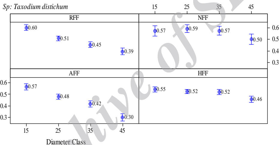
شکل ۵. تغییرات در طبقات قطری روش‌های واقعی (RFF)، طبیعی (NFF)، مصنوعی (AFF) و هوندادل (HFF) برای دارتالاب (اعداد ذکر شده در پانل‌ها میانگین ضرایب در طبقات قطری است)
