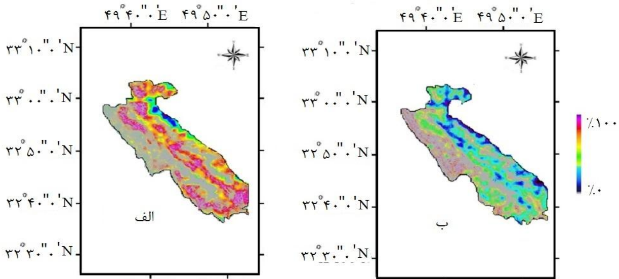
شکل ۲. نقشه تکه‌تکه‌شدگی تولید شده از روش: الف) انترویی و ب) پیوستگی
